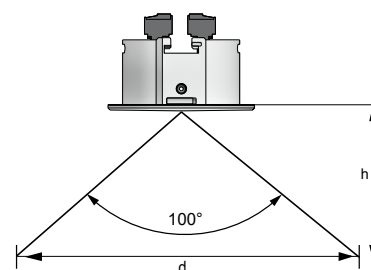
取り付け高さ／カバー範囲 LDALI-MS4-BT
